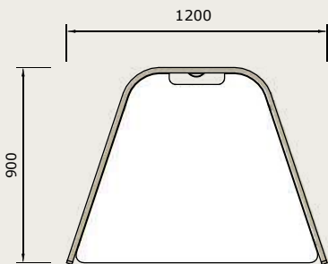
01 PLAN 1:15
