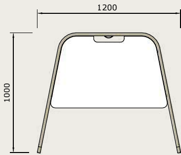
01 PLAN 1:15
