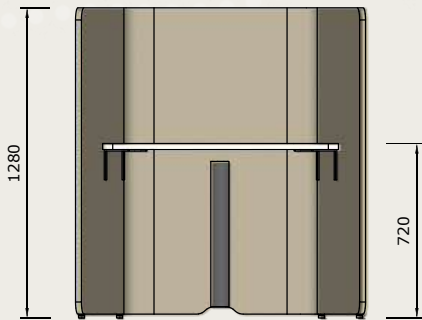
02 FRONT ELEVATION 1:15
