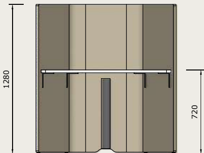
02 FRONT ELEVATION 1:15
